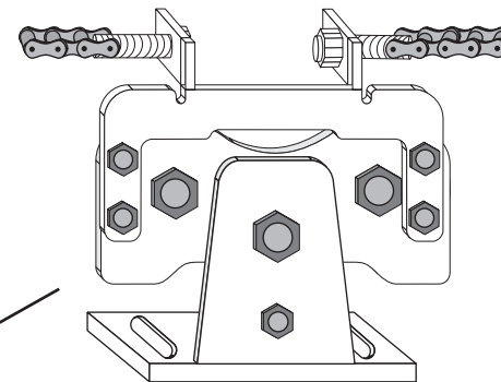
主動板 ACTIVE BRACE
