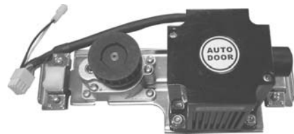
直流無刷馬達及減速齒輪組 BRUSHLESS DC MOTOR
