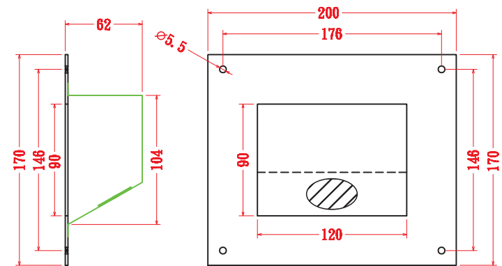
實際尺寸圖
