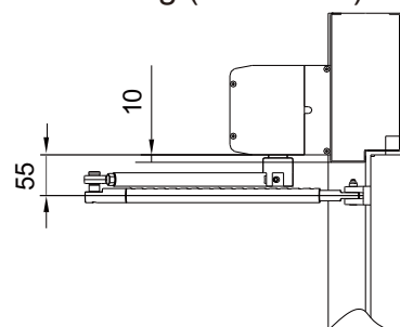
外推式開門方向 (右側開門) Mounting (eg. for Right Open, Top View)
