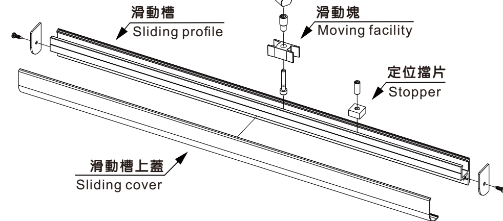
內拉式滑槽示意圖
