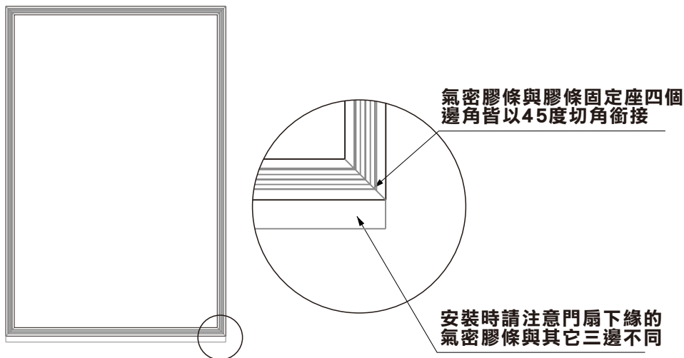
氣密膠條安裝方式
