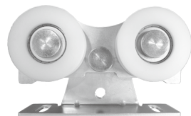
吊輪組 4 組 HANGING TWIN WHEEL-4PCS
